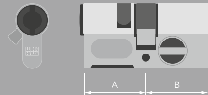
Profil-Doppelzylinder Typ BO 05 (einseitig elektronisch kontrolliert)
